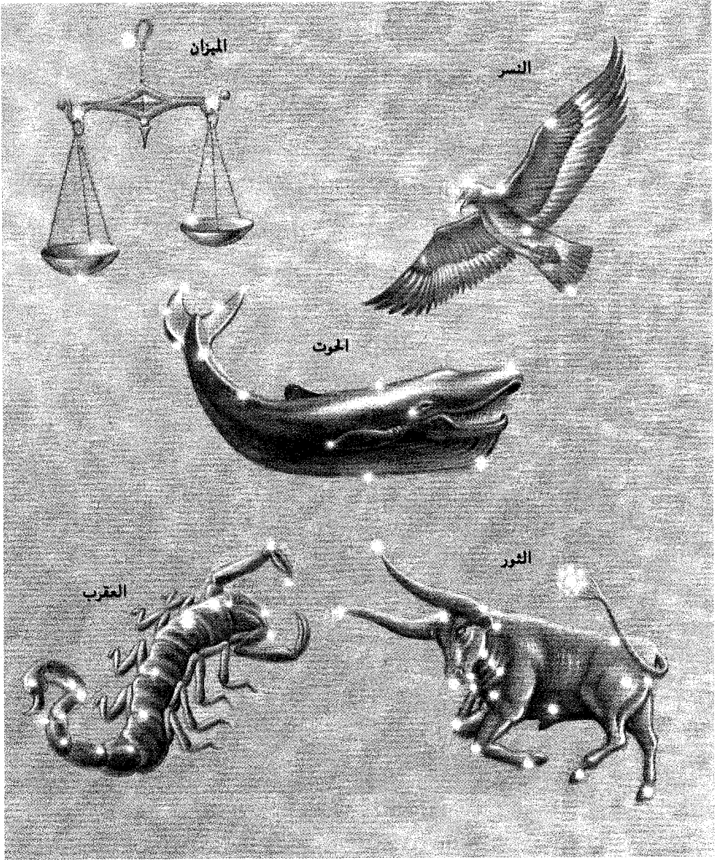
شكل (110) يوضح بعض الهيئات التي ترى عليها بروج السماء
