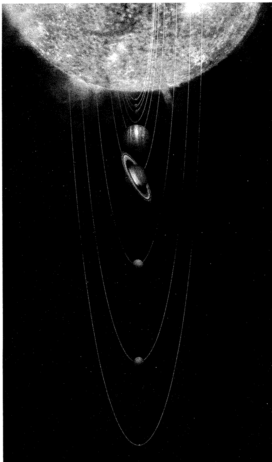
رسم للمجموعة الشمسية ومداراتها حول الشمس، وحجم كل منها بالنسبة لها. - الشمس - عطارد - الزهرة - الأرض - المريخ - المشترى - زحل - يورانيوس - نبتون - بلوتو
