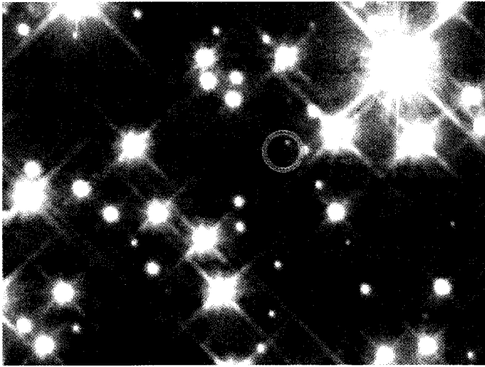
شكل (83) صورة للتجمع النجمي (WFPC 2 ) يضم في داخل الدائرة الخضراء أحد النجوم النايضة
