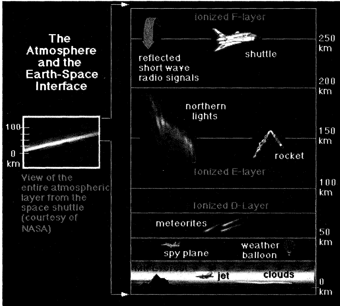
شكل (99) يوضح بعض نطق الغلاف الغازي للأرض
