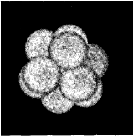
شكل (106) يوضح شدة الترابط في داخل نواة ذرة الكربون ( ^{11}10 ملليمتر)
