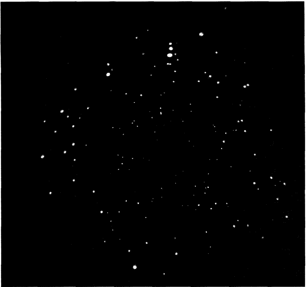
شكل (114) صورة توضح بقايا انفجار المستعر الأعظم قبيلا وما حوله من كوكبات
