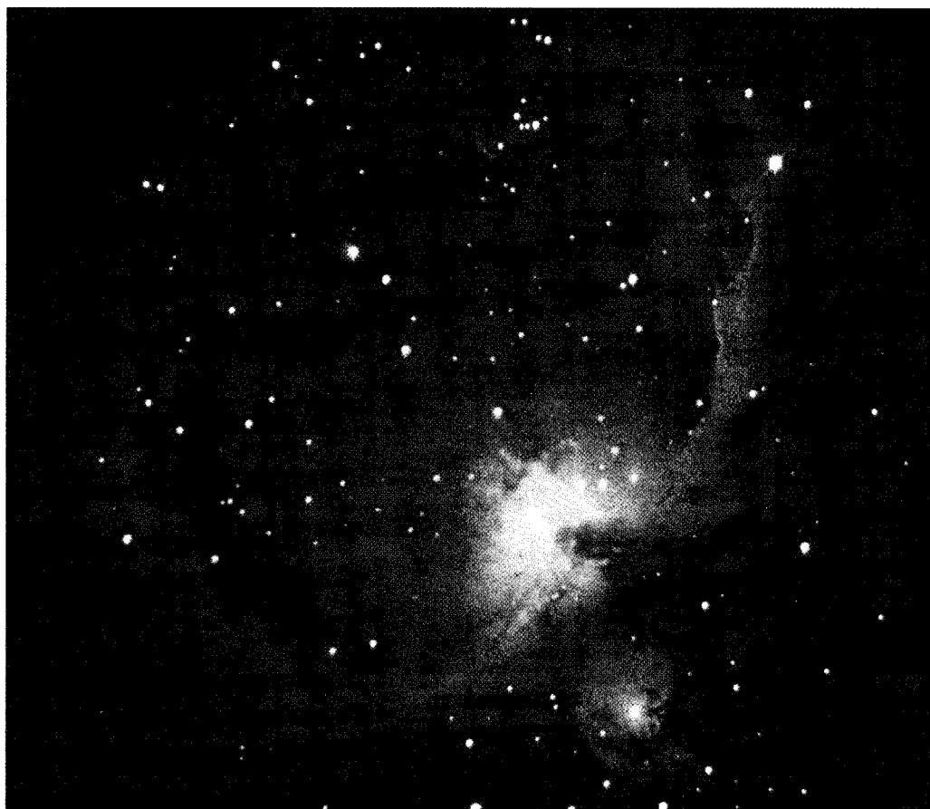
شكل (22) صورة حقيقية لدخان كوني تناثر من جراء انفجار نجم من نجوم السماء
