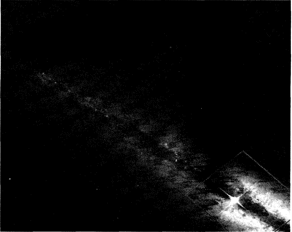
شكل (87) صورة للمجرة (NGC 4013) في الضوء المرئي
