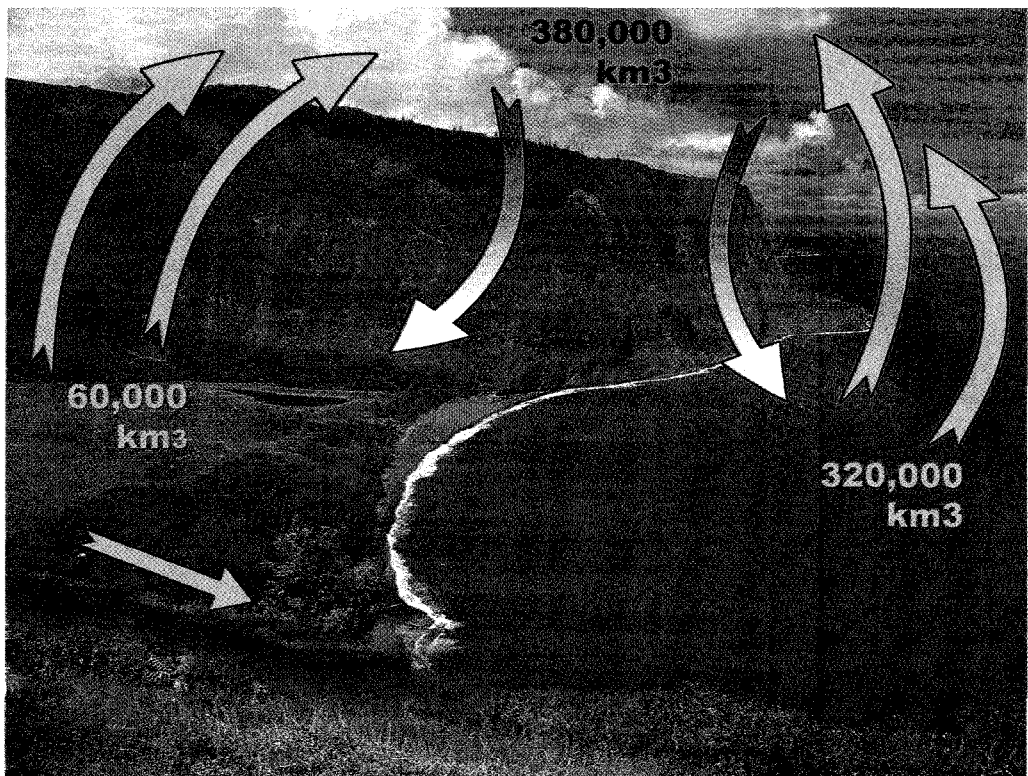
شكل (93) رجح ماء الأرض إليها عبر دورة الماء حول الأرض بكميات متساوية ما بين التبخر وهطول الأمطار
