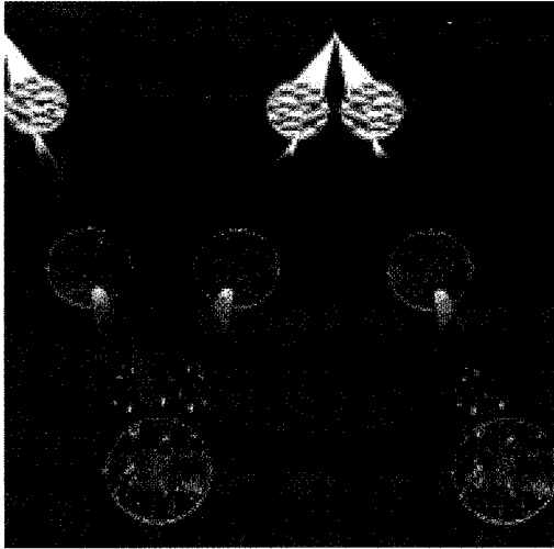
شكل (43) يوضح عمليتي الانفجار العظيم والانسحاق الشديد للكون وإعادة خلق أرض غير الأرض وسماوات غير السماوات.
