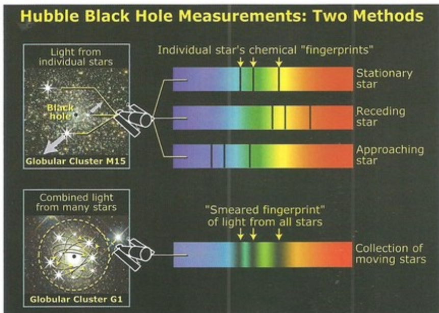
شكل (63) يوضح قياس تليسكوب هابل للنجوم الخائسة الكانسة بواسطة قياس تباعد النجوم المجاورة أو اقترابها منها بظاهرة الحيود إلى أي من الطيفين الأحمر أو الأزرق
