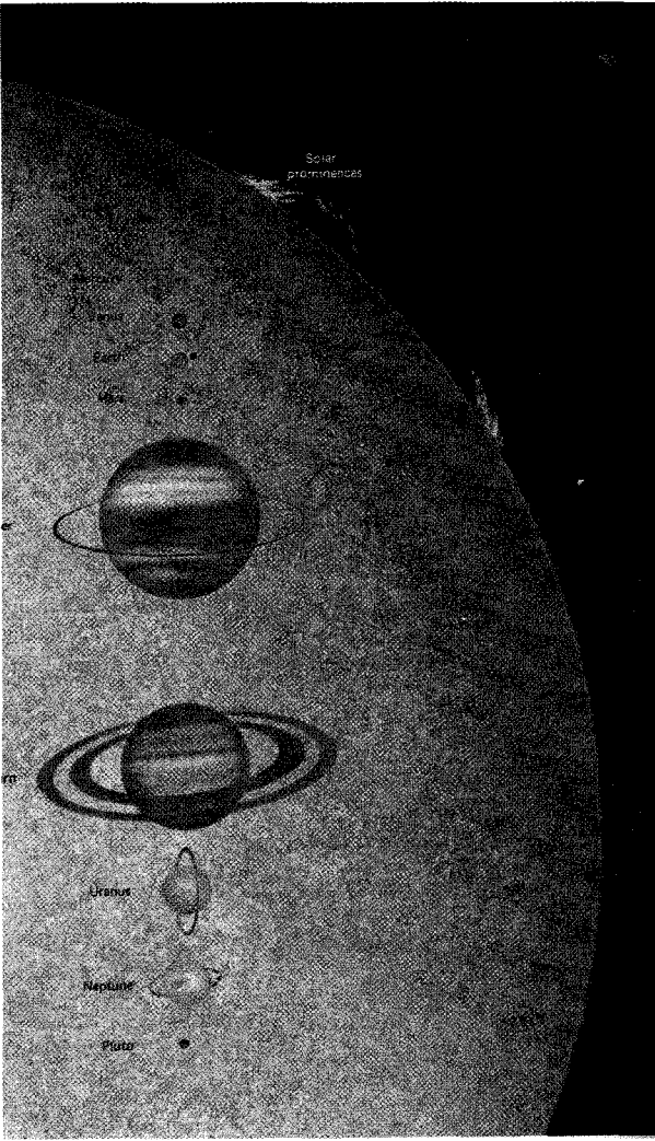
شكل (117) يوضح حجم كواكب المجموعة الشمسية بالنسبة إلى الشمس
