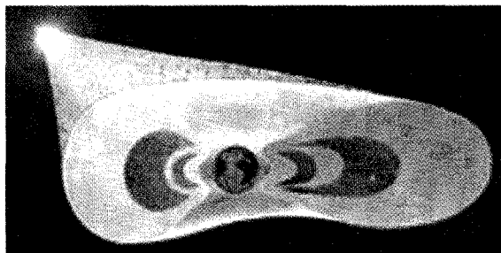
شكل (98) يوضح نطق الإشعاع من الغلاف الغازي للأرض
