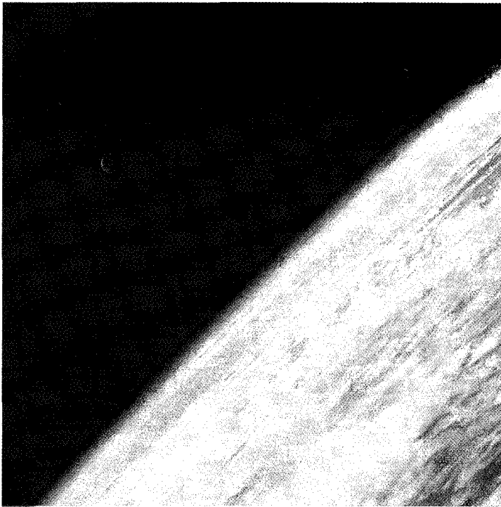
شكل (78) يوضح رقة طبقة النهار في نصف الأرض المواجه للشمس بسبب لا يتعدى 200 كم وباقي الكون ظلام دامس
