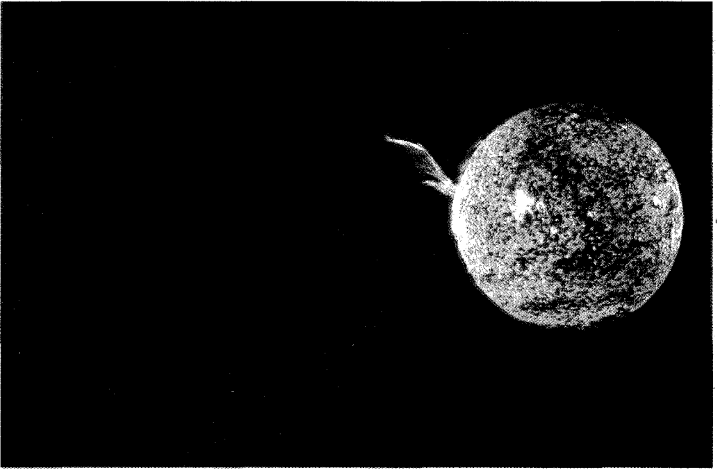
شكل (152) يوضح إحدى الانفجاعات الشمسية الكبيرة التي صورتها عدسات مختبر السماء أشعة لاب
