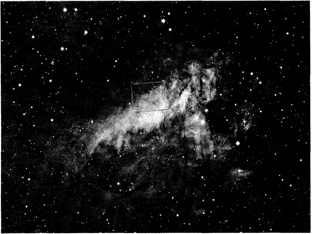
شكل (88) صورة للسديم (WFPC 2 ) أخذها المرصد الإنجليزي الأسترالي
