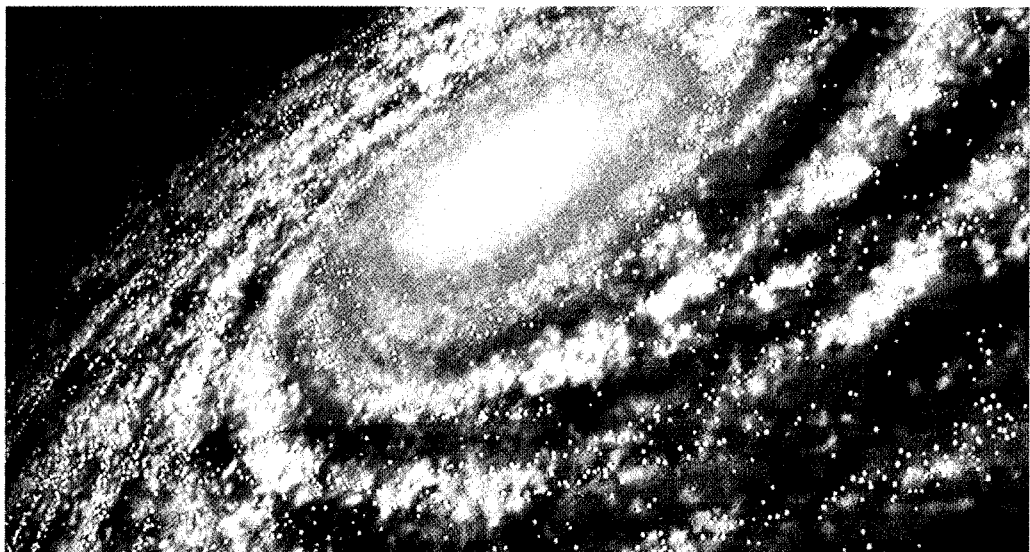
شكل (30) صورة لقرص إحدى المجرات الحلزونية الضخمة
