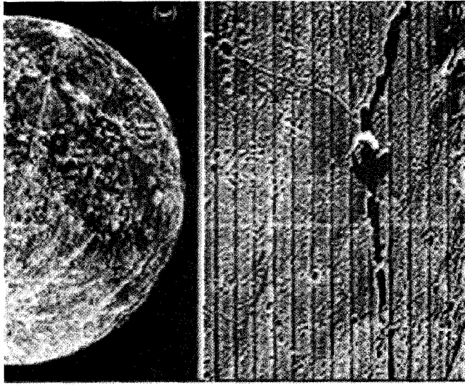
شكل (164) صور لشقوق في القمر
