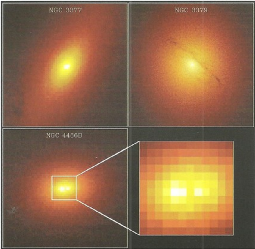
شكل (71) يوضح صوراً متفرقة لنجوم خانسة كائسفة في قلب عدد من المجرات المختلفة
