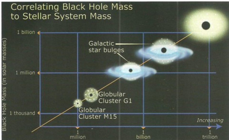
شكل (62) يوضح تقدير كتلة النجم الخائس الكانس بمقارنته بكتل النظم النجمية
