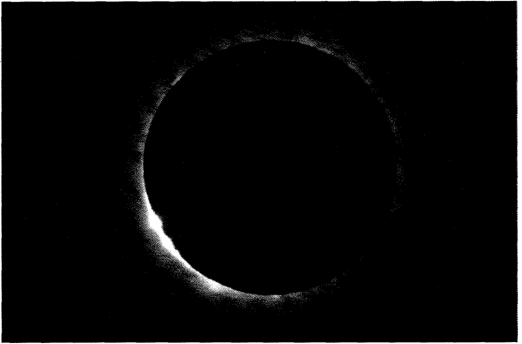
شكل (156) توضح الكسوف الكلي للشمس.
