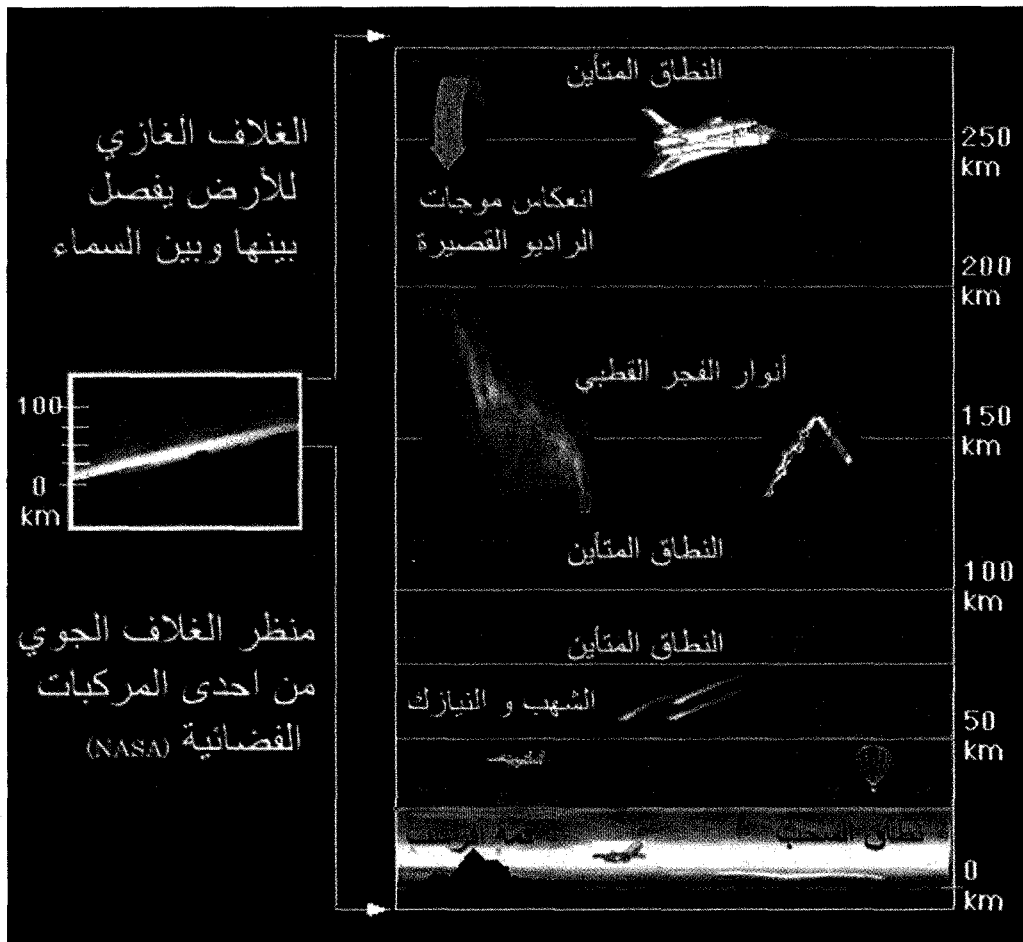
شكل (136) يوضح نطق الغلاف الغازي للأرض
