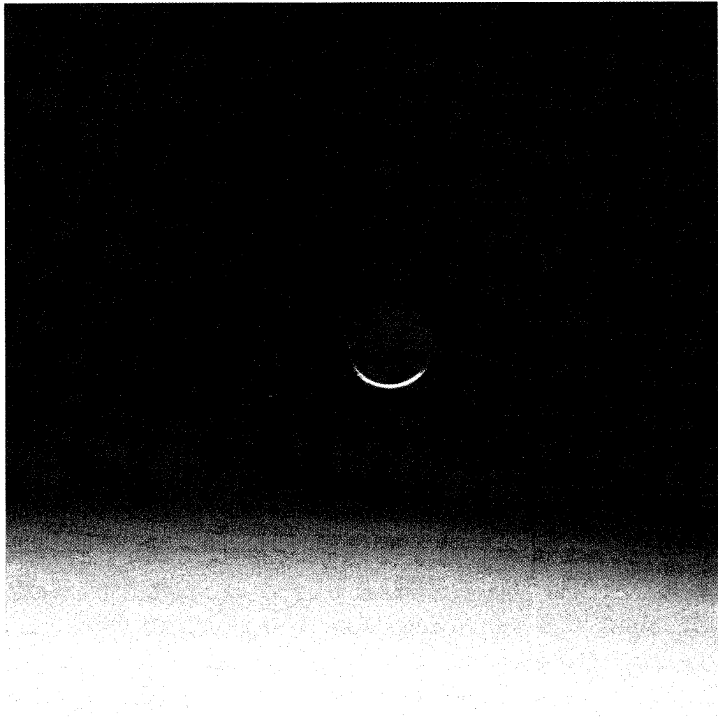
شكل (168) يوضح ظلمة الكون خارج نطاق الغلاف الغازي الملامس للأرض ورقة طبقة إنارة القمر لسطح الأرض بالليل
