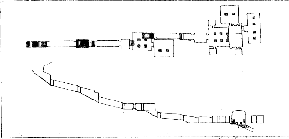
٦٦ - مسقط أفقى ورأسى لمقبرة الملك سيني الأول .
