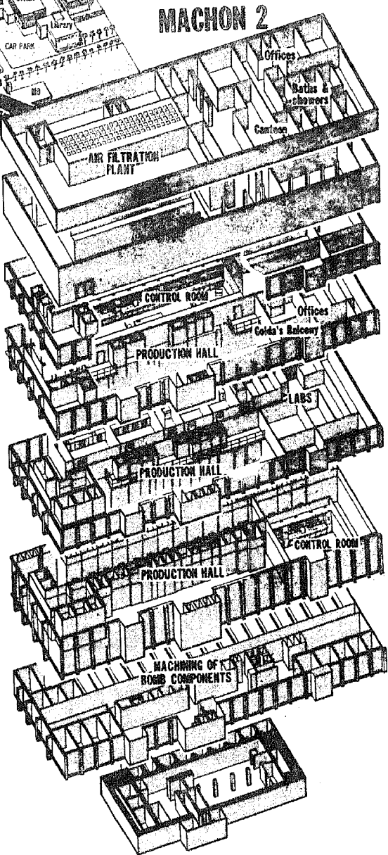
مخطط توضيحي لمفاعل ديمونا من الخارج والطوابق الستة الموجودة في باطنه
