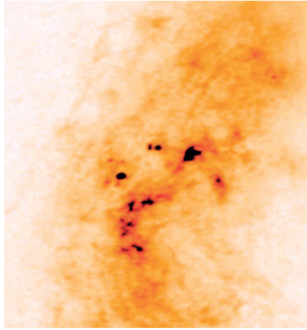
مجموعة مرصد «ألما» ترى الكتل الغازية المكونة للنجوم في الحجر (الجدار).
