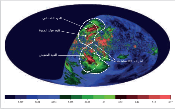
فيزياء الفلك
