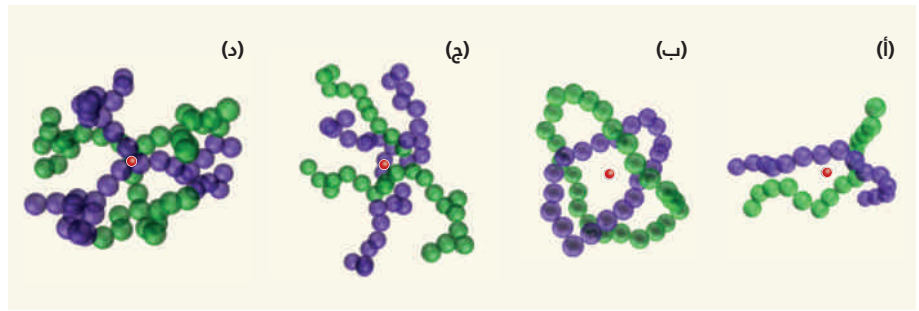
الشكل 1 | جسيمان .. مركز واحد. «د» - «أ»: يمكن للجسيمات اللينة المُشكَّلة من البوليمرات أن تتغير شكلها، وأن تتداخل بحيث تتطابق مراكز كتلتها، كما هو معروض هنا لأزواج من سلاسل البوليمر «أ»؛ وحلقات البوليمر «ب»؛ ونجوم البوليمر ثلاثية الأبعاد «ج»؛ والشجرية أو النجوم المتصلة في «د». تتطابق مراكز الكتل (النقاط الحمراء) للجسيمات الخضراء والأرجوانية، حتى في حالة عدم تداخل جميع وحدات بوليمرية (monomers). (الرسوم مهداة من لورينزو روفجاتي)
