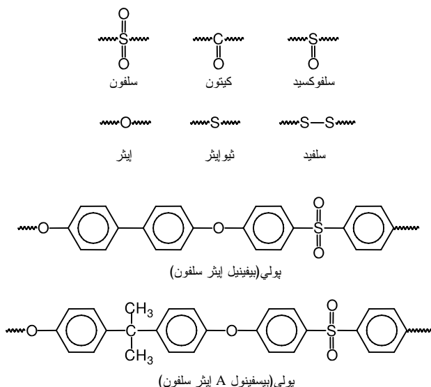
الشكل (1-7): الزمر الوظيفية وكتل بناء أنماط من پولي (إيثر سلفون)
