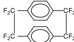
ثماني فلورو [2.2] پارا سيكلوفان
