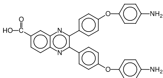
حمض 3-3' بيس (4- أمينو فينيل أوكسي فينيل )- كينوكزالين -6- كربوكسيليك
