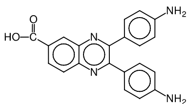
حمض 3-3' بيس (4- أمينو فينيل )- كينوكزالين -6- كربوكسيليك
