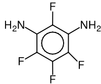
3،1-ثنائي أمينو رباعي فلوروبنزين
