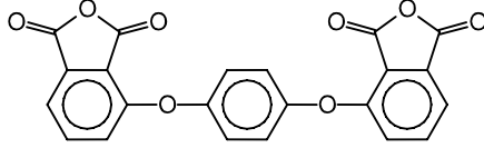
ثنائي أنهيدريد 3،1-بيس (3،2-ثنائي كربوكسيل فينوكسي) - بنزين
