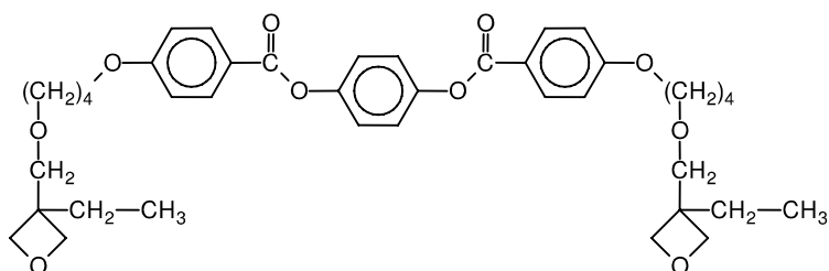
حمض بنزويك، 4-(3-إيثيل -3-أوكسيبتانيل) ميثوكسي [بوتوكسي] -4،-4-فينيلين إستر
