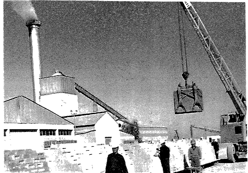
● مصنع الطابوق
