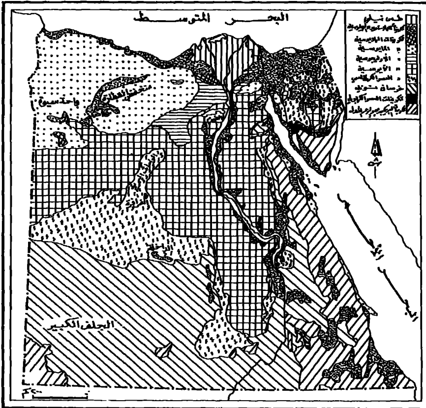
التكوين الجيولوجي
