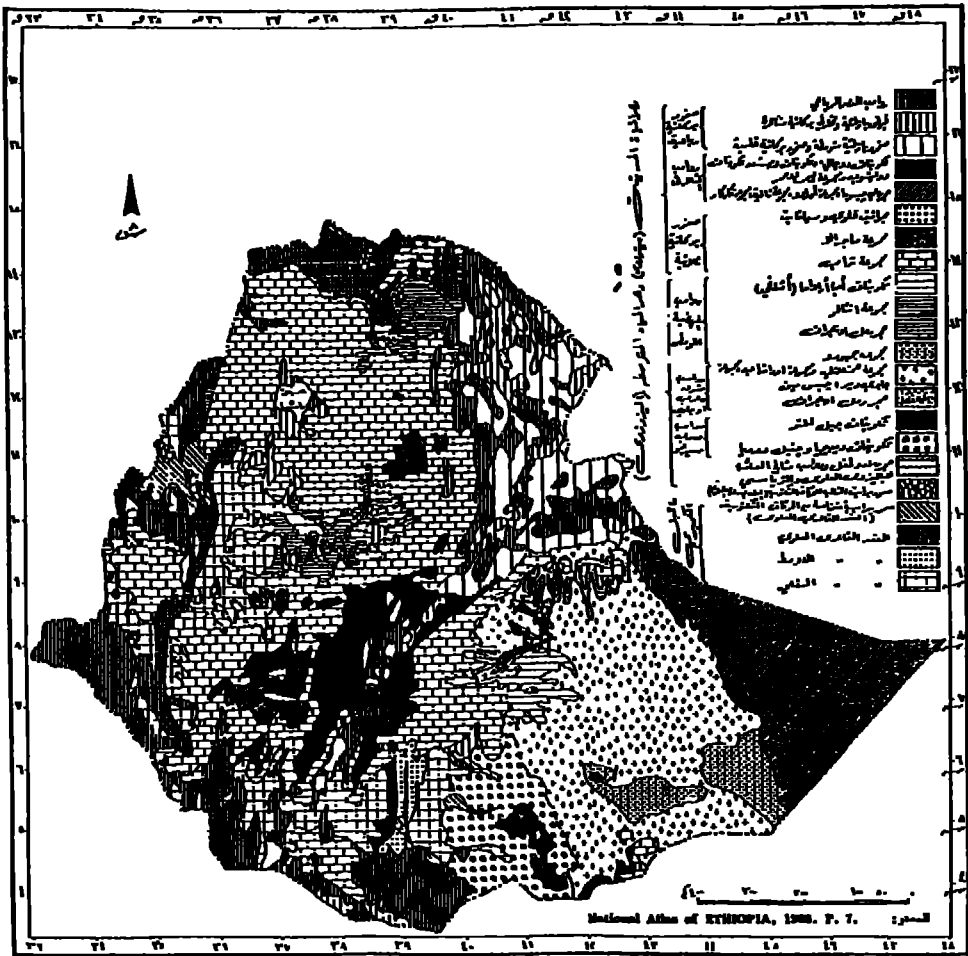
جيولوجية اثيوبيا
