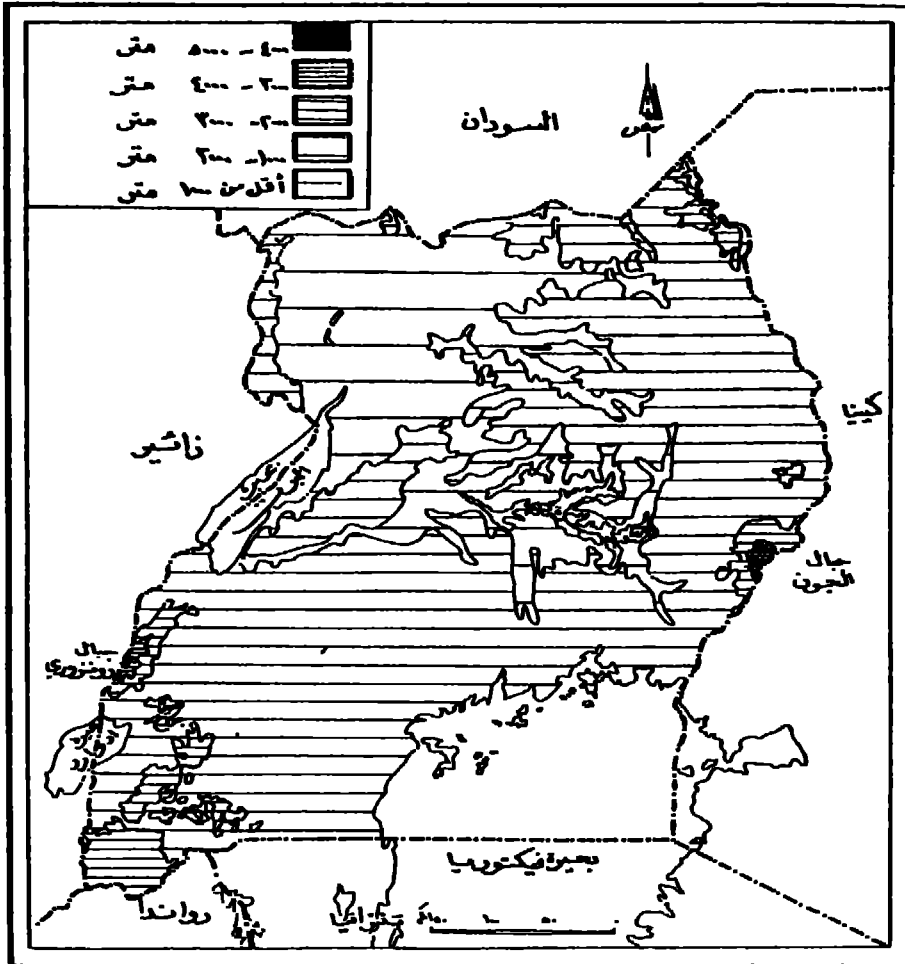
سطح الأرض
