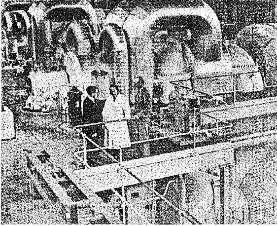
صالة التربينات ، بمحطة انتاج الكهرباء من الذرة ، بكلدهول بانجلترا ، وهي تربك التربينات الهائلة التي يديرها البخار فتدور في حقولها المغناطيسية ، فنتج من ذلك الكهرباء . وتنتج التربينة الواحدة منها ٢٣٠٠٠ كيلوواط
