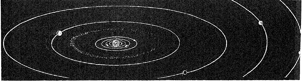
شكل ابصاحي لمجموعةتنا الشمسية: الشمس في الوسط ، يليها عطارد، فالزهرة ، فالارض ، فالمرخ . فالكوكب الذي تطعم . فالشترى . فزحل . فاورانوس . فبتون فبلوتو
