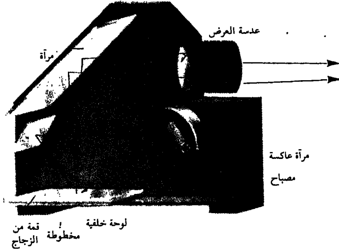
جهاز عرض الصور المعتممة «الايكوب»
